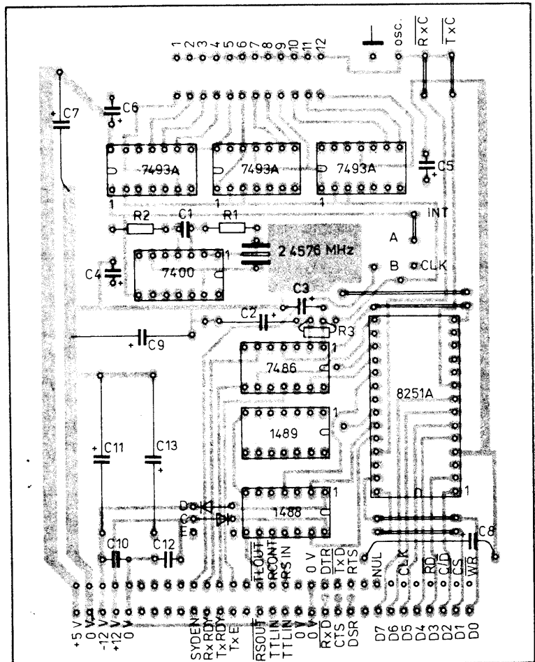
Obr. 10. Rozložení součástek na desce s plošnými spoji interfejsu RS-232C W002
